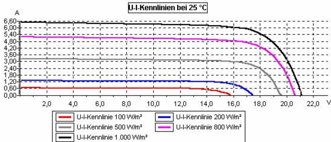
Bild 3 U-I-Kennlinienfeld
